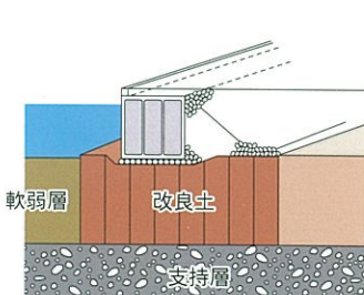
河川築堤、護岸等の基礎
