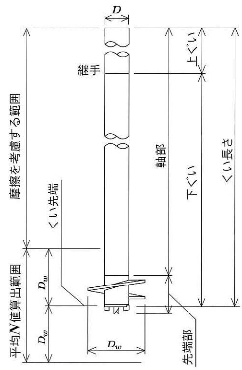
各部名称(押込み方向)
