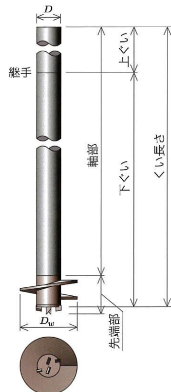
各部名称
